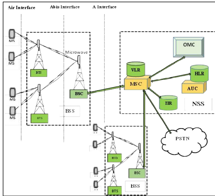
Fig. 2. GSM overview
